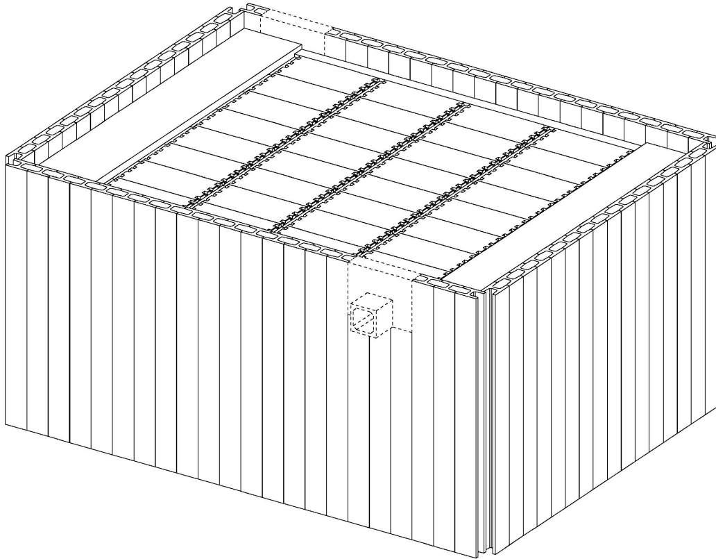
【背面斜視図】
